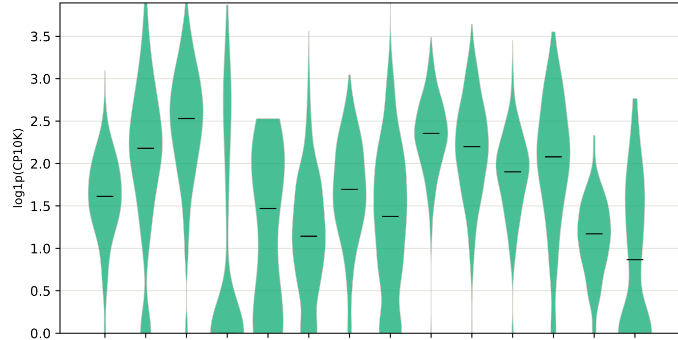
CLDN4
