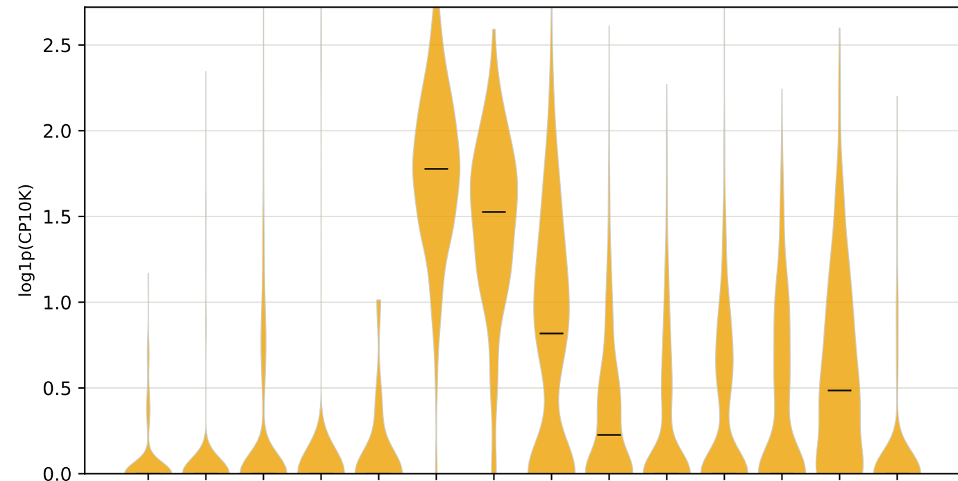
SFN
